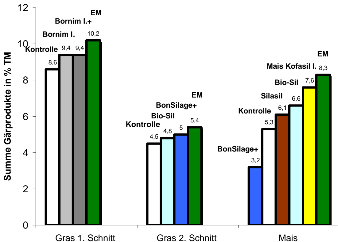
Abb. 3: Einfluss von unterschiedlichen Zusätzen auf die Summe gemessener Gärprodukte in den Silagen nach 90 Tagen
