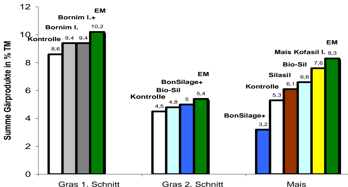
Abb. 3: Einfluss von Zusätzen auf die Summe gemessener Gärprodukte in den Silagen nach 90 Tagen
